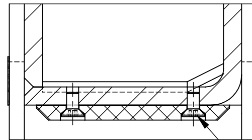
SECTION B-B SCALE 1 : 2
