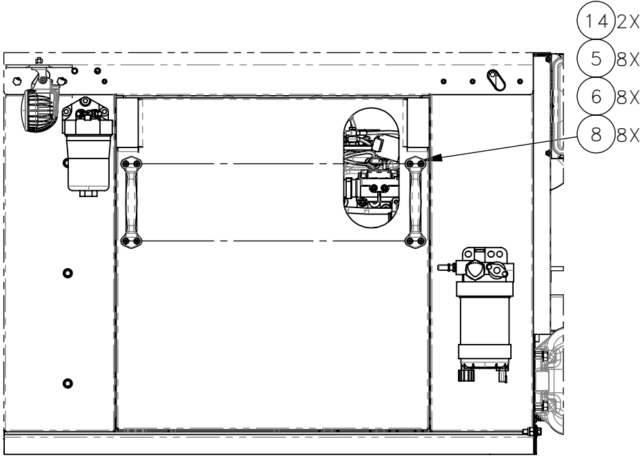
SECTION D-D 2 DOORS QTY'S PER DOOR
