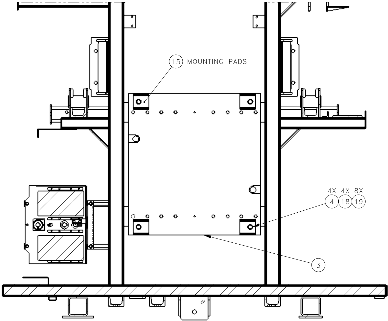
SECTION A-A
