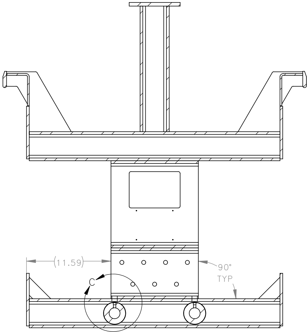
SECTION A-A SCALE 1 : 8
